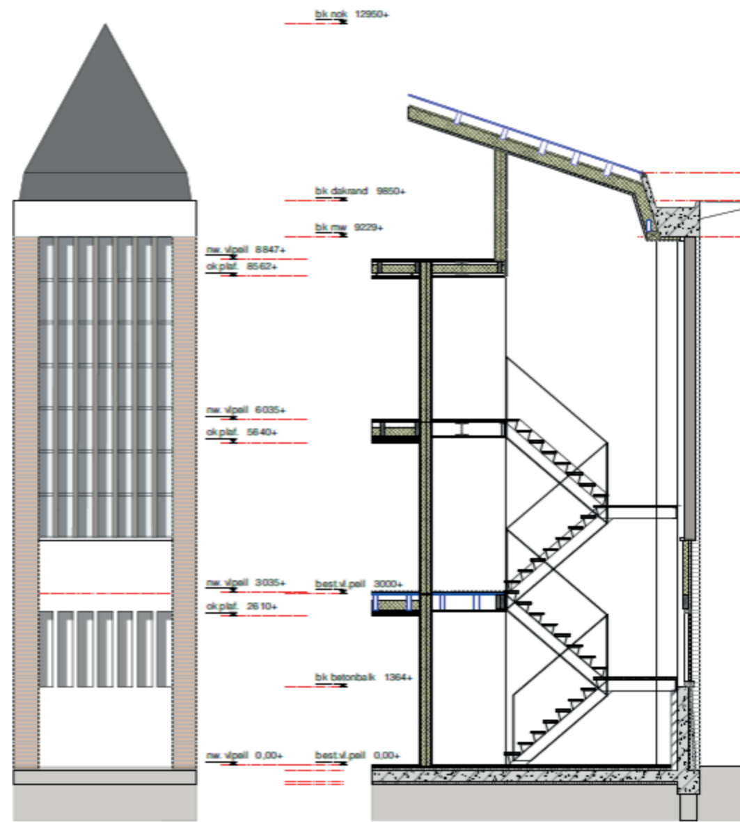
Gevelfragment J
