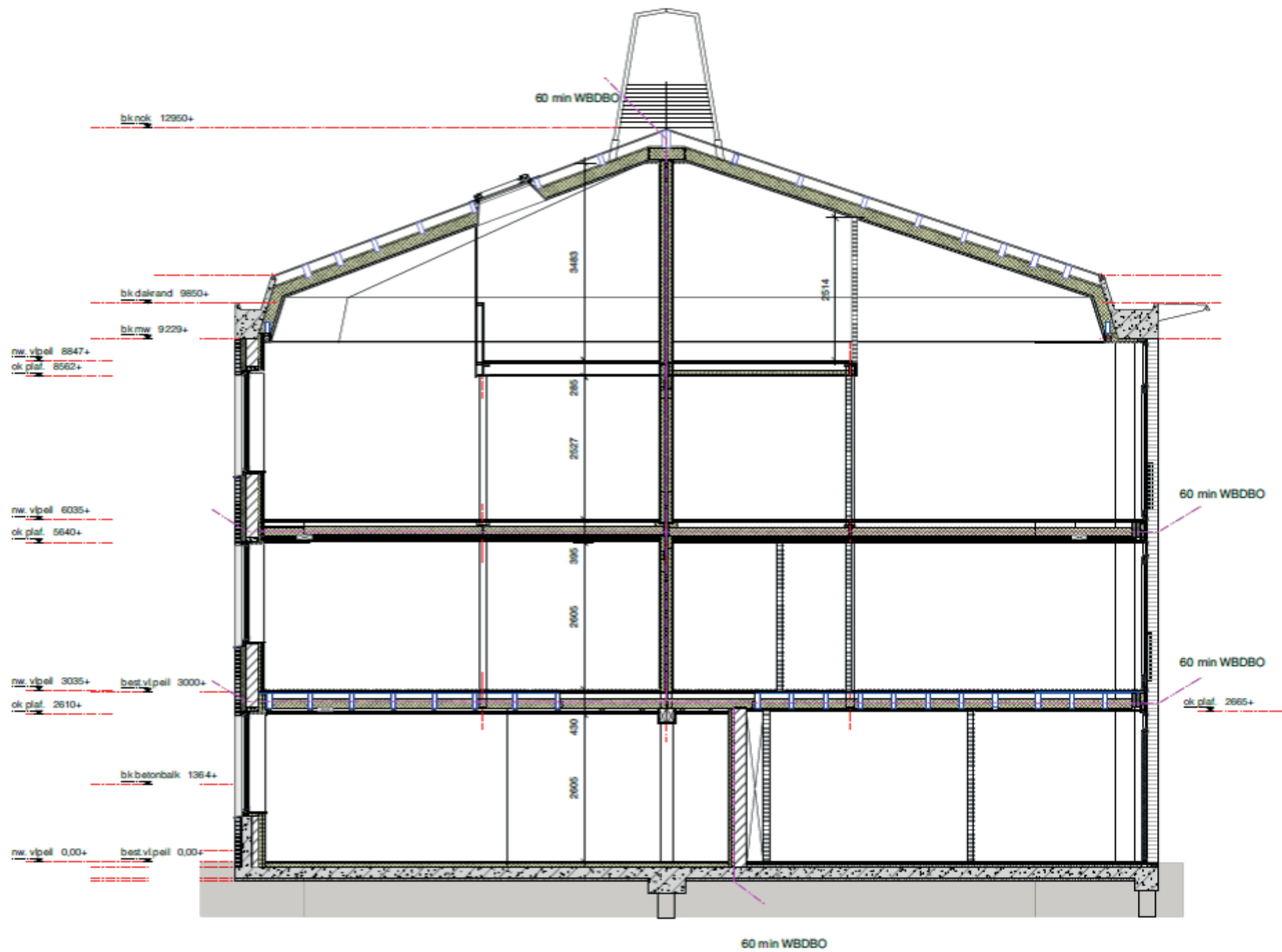
DOORSNEDE X-X
